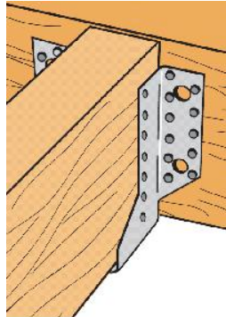
SAE sur bois - clouage complet
