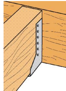
Fixation sur support BOIS - Clouage complet
